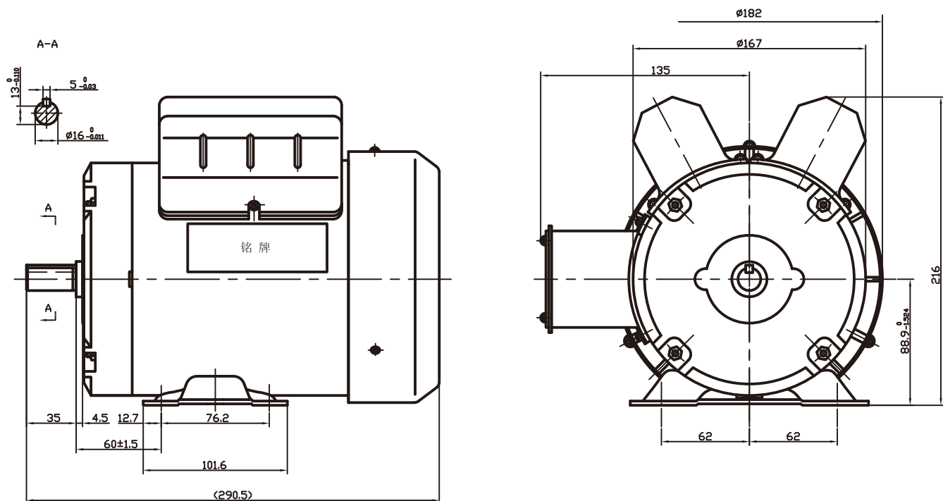
YCYN5652D-1外形图
