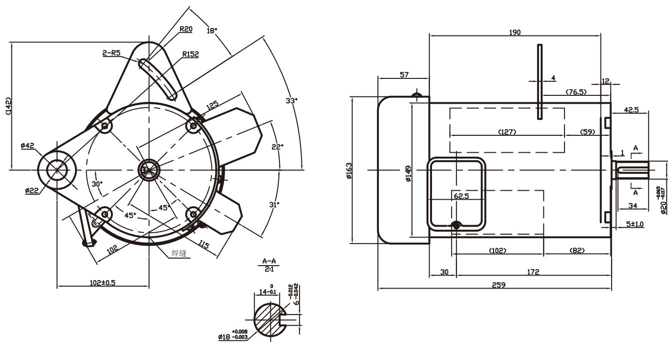
YCYGL8052外形图
